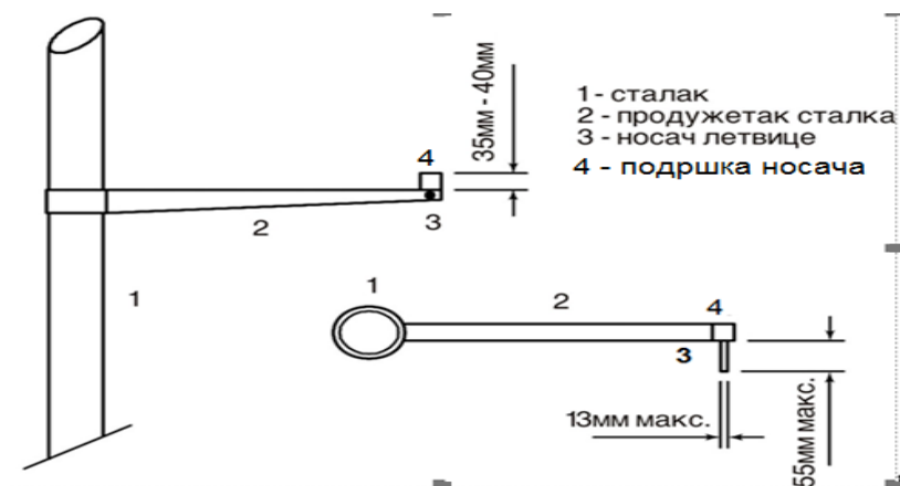
Скица 8 - Сталци за скок мотком
