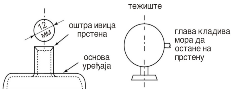
Скица 20. Уређај за контролу тежишта главе кладива
