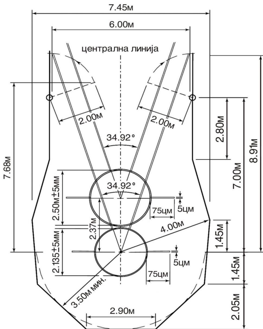
Скица 24. Заштитна мрежа са одвојеним круговима за бацање диска и кладива.
