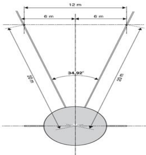
Одређивање сектора са углом 34,92^\circ
